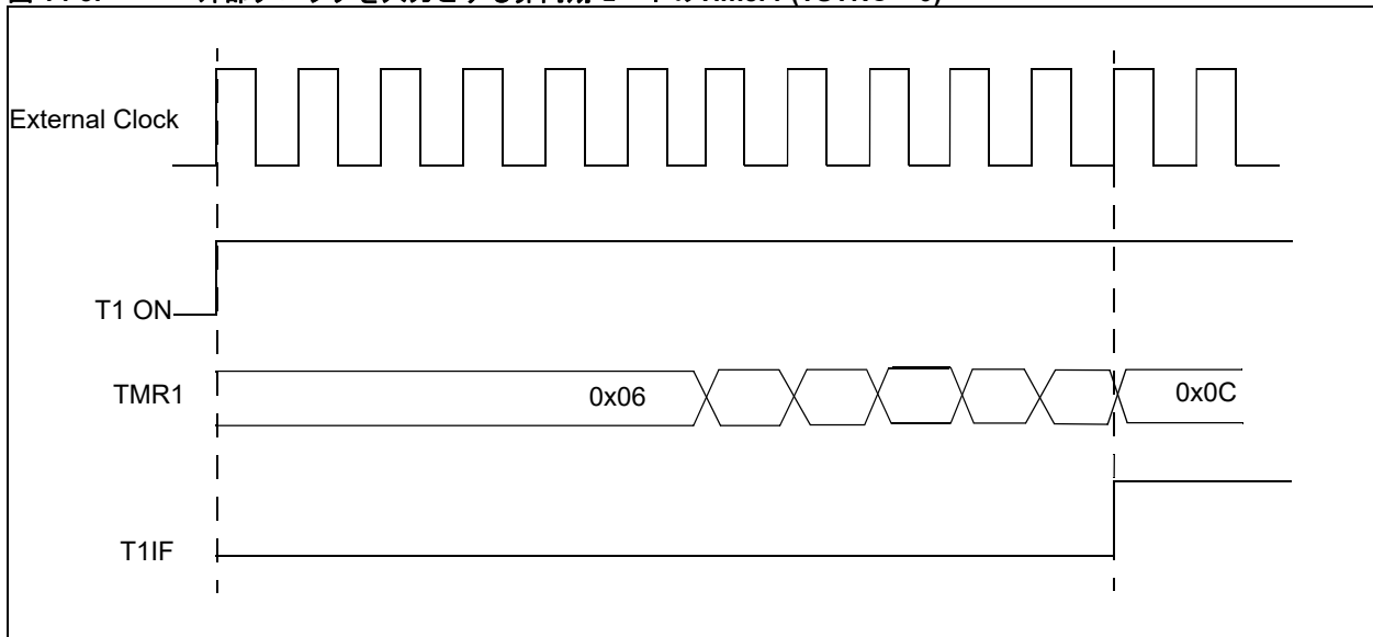
図 14-5: 外部クロックを入力とする非同期モードのTimer1 (TSYNC = 0)
