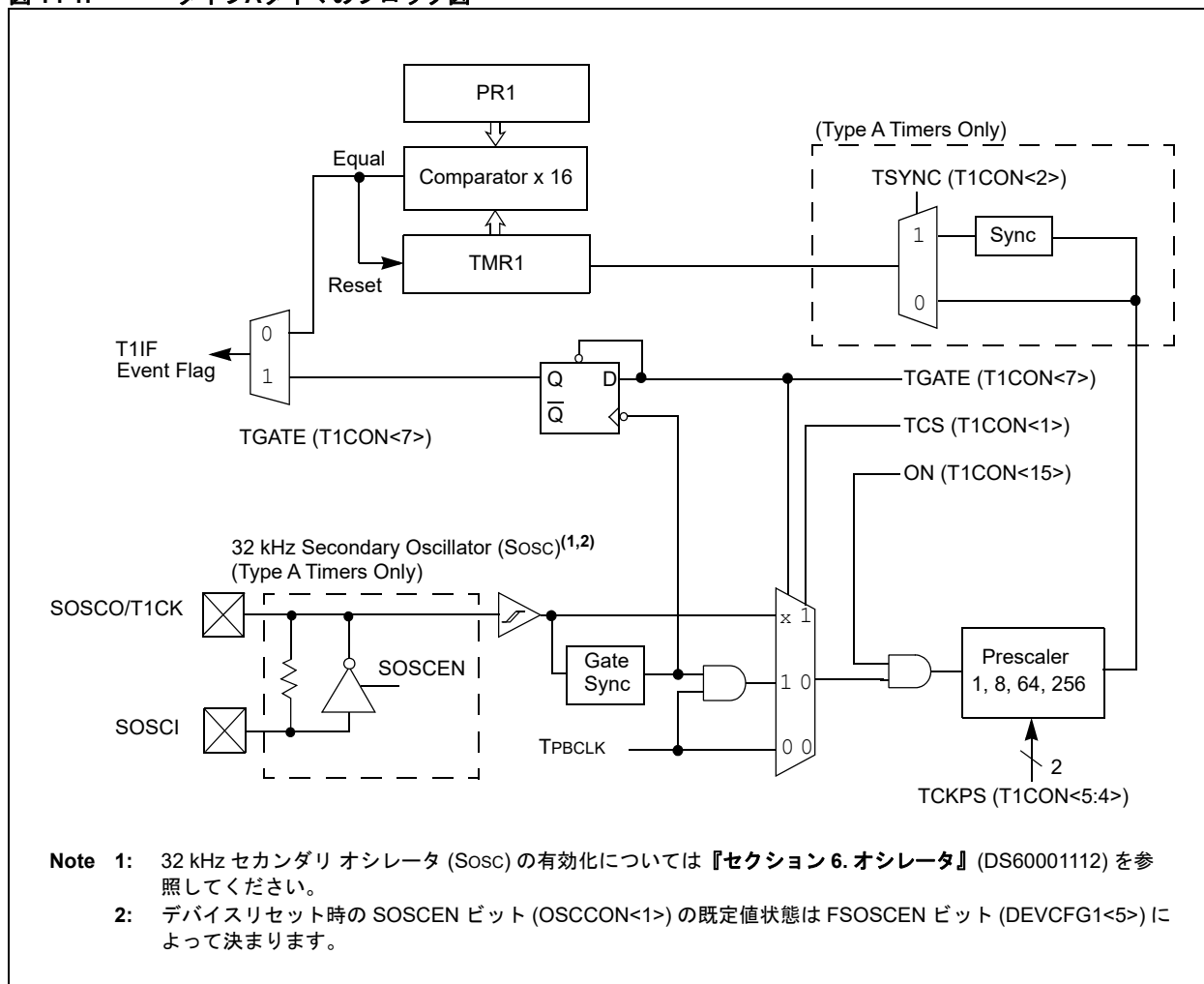
図 14-1: タイプ A タイマのブロック図
