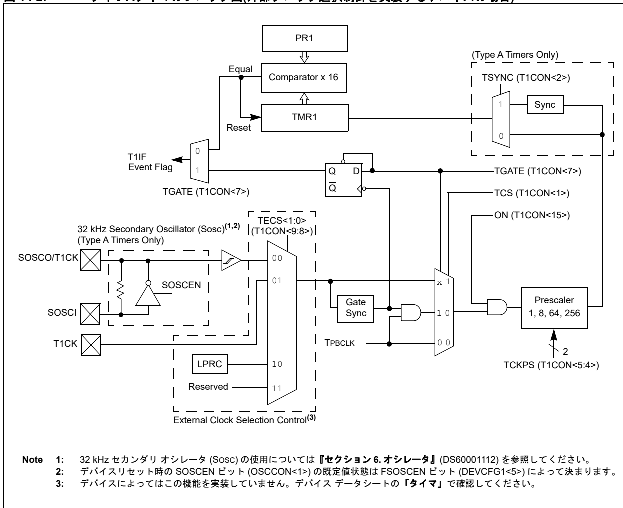
図 14-2: タイプAタイマのブロック図(外部クロック選択制御を実装するデバイスの場合)
