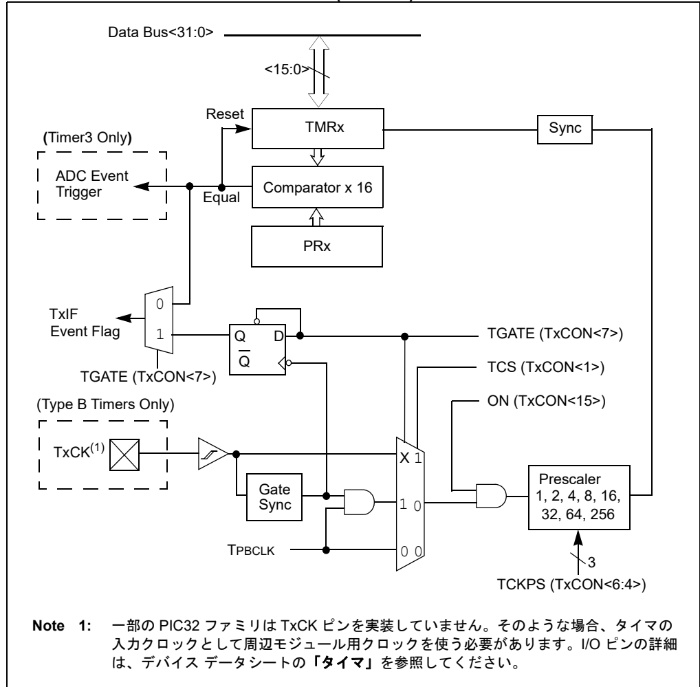
図 14-3: タイプ B タイマのブロック図 (16 ビット)
