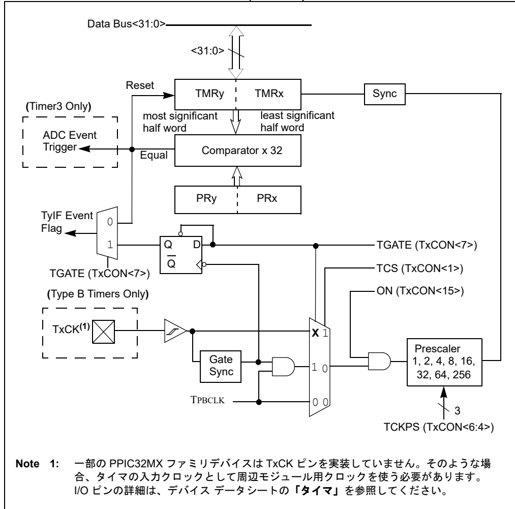
図 14-4: タイプBタイマのブロック図(32ビット)
